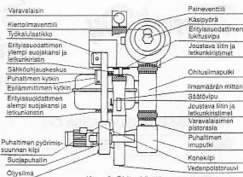
Kuva 2. Ohituskäyttö
