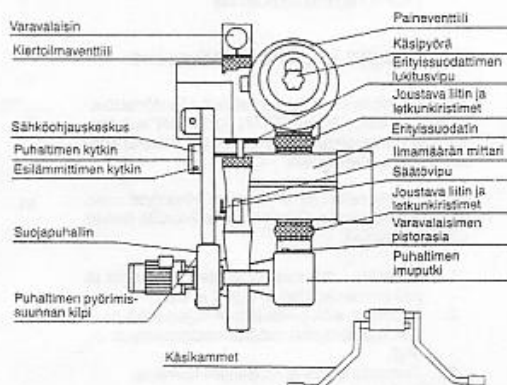
Kuva 3. Suodatuskäyttö
