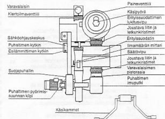
Kuva 3. Suodatuskäyttö
