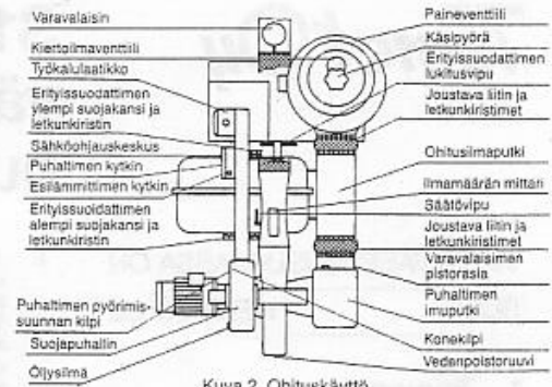
Kuva 2. Ohituskäyttö
