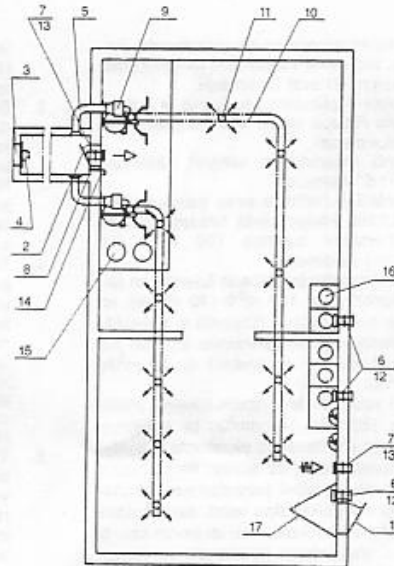
Kuva 1. S1-luokan väestönsuojan laitesijottelu- ja laitteistoluetelo
