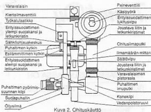
Kuva 2. Ohituskäyttö
