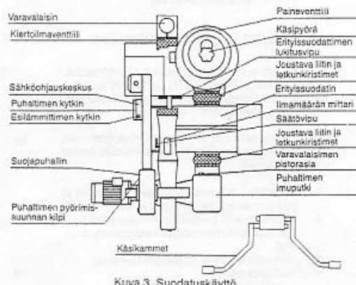
Kuva 3. Suodatuskäyttö
