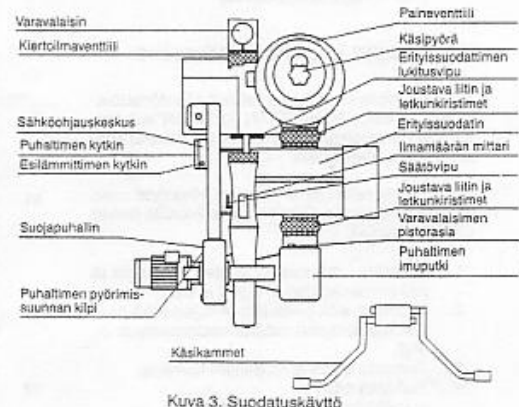
Kuva 3. Suodatuskäyttö
