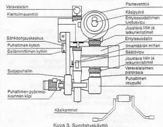
Kuva 3. Suodatuskäyttö
